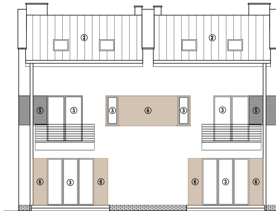
ELEWACJA TYLNA / OGRODOWA
