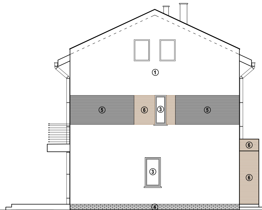
ELEWACJA BOCZNA
